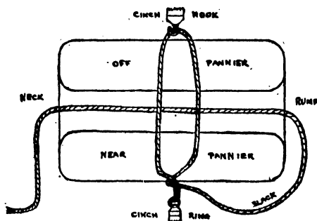
LONE JACK HITCH, FIG. 1
